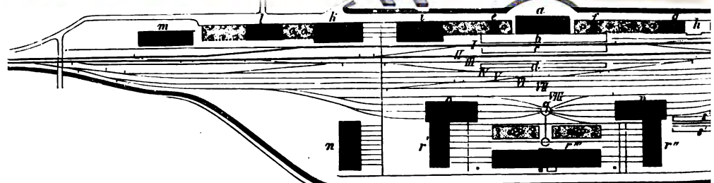
23. Aanleg van een spoorwegstation.
