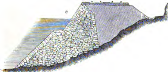
11a. b. c. d. Onderbouw en aardebaan.
