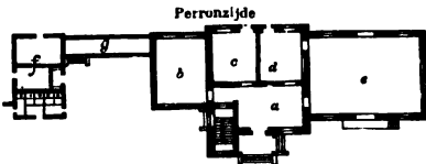
6b. Grondvlak van het tussenstation.
