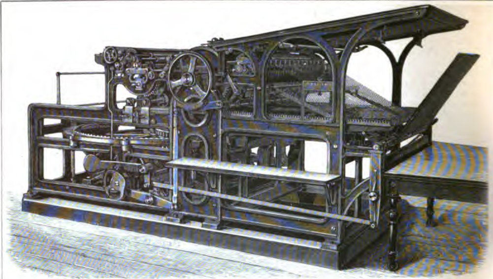
1. Snelpers met cirkelbeweging en versterkte inktrollen (König u. Bauer).
