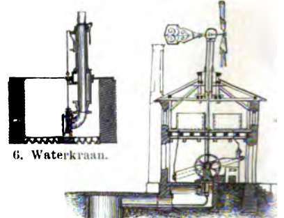
7. Waterstation met windmolen.
