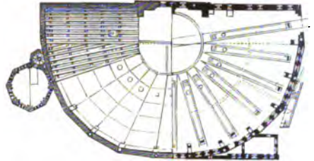
5. Grondvlak der locomotievenloods.
