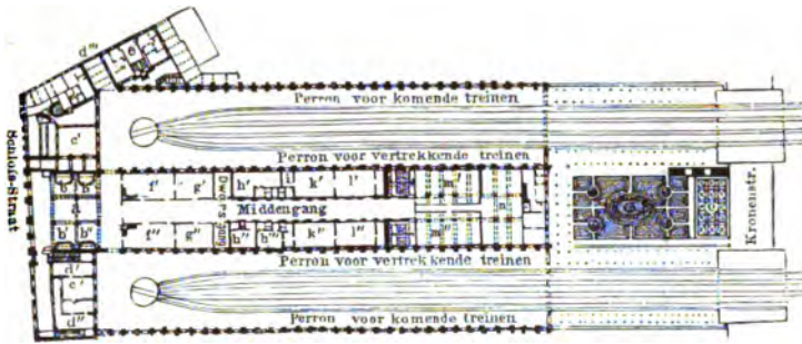
1. Grondvlak van het stationsgebouw te Stuttgart.
