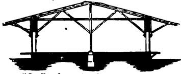
26. Goederenloods, doorsnede.
