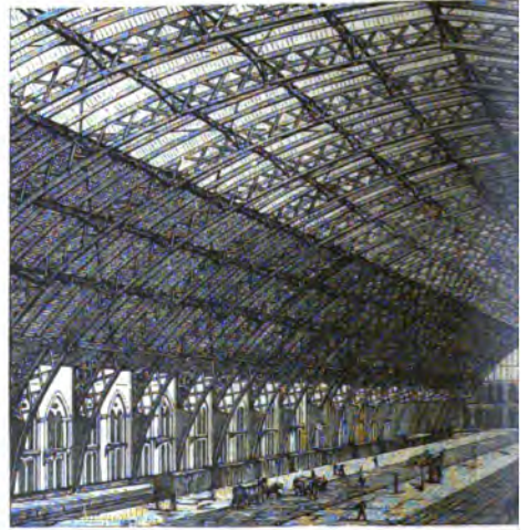
11. IJzeren dak met boogvormig traliewerk (Get
