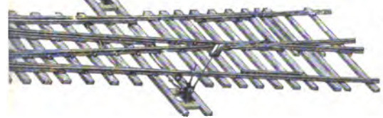
18. IJzeren bovenbouw op overlangsche liggers, drie-delig systeem.
