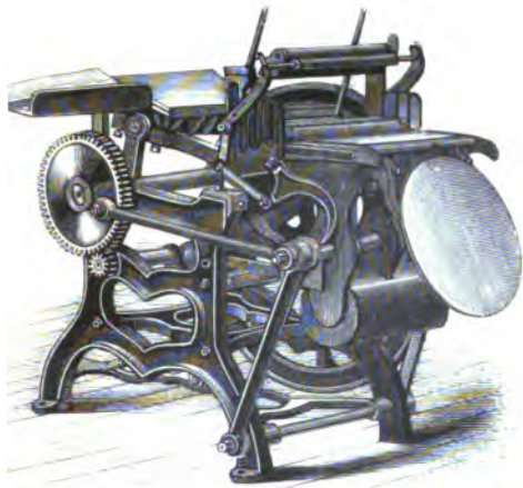
liberty-degeldruksnelpers van Weiler (A. Waldow).
