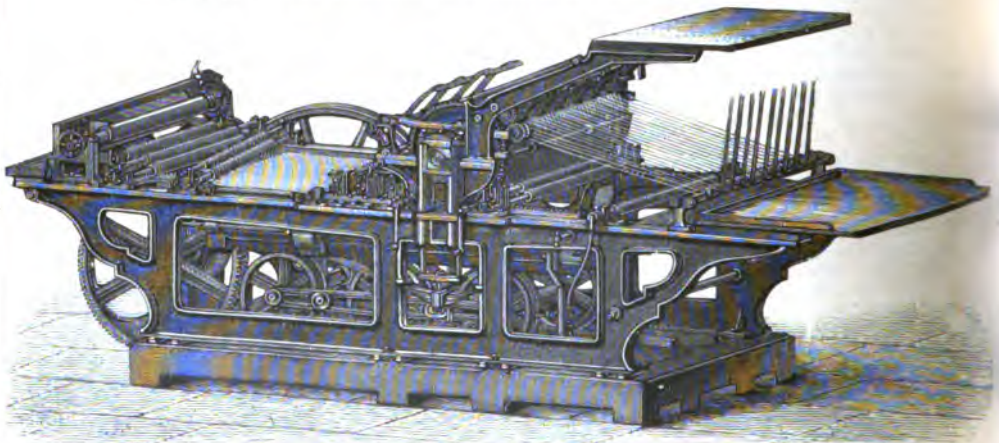
6. Steedruksnelpers (Schmiere, Werner u. Stein).
