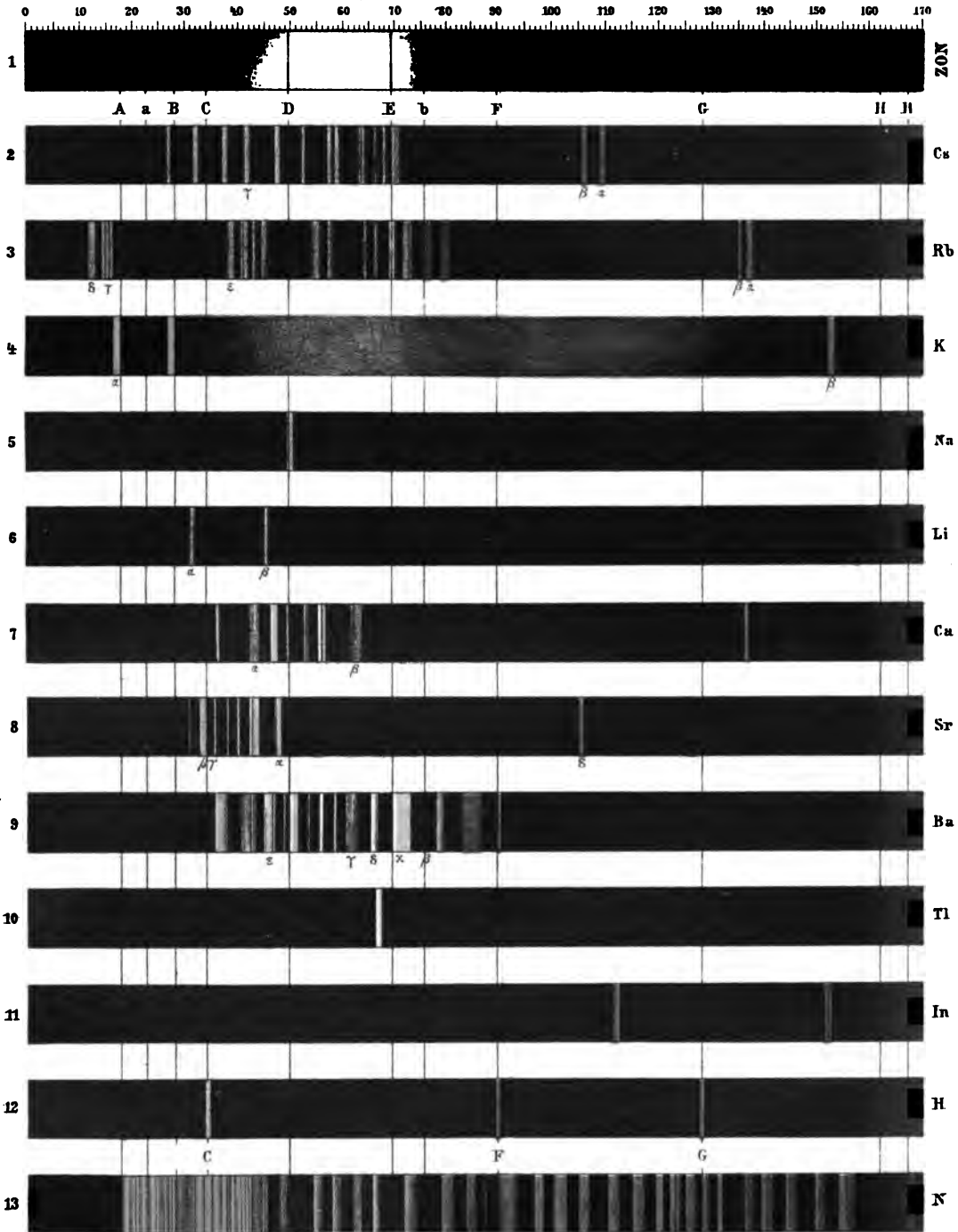
1. Zonnespectrum. 2-11. Spectra van verschillende metalen. 12. Waterstof. 13. Stikstof.
