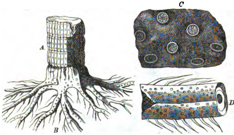
Fig. 2. A. Sigillariastam . B. De wortel, stigmaria geheeten. C. Een stuk stigmaria in natuurlijke grootte. D. Zulk een stuk verkleind.
