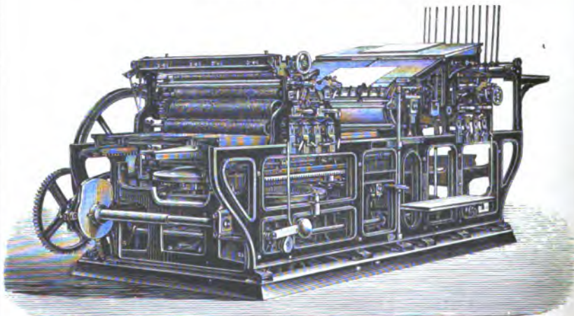
4. Snelpers voor het drukken met twee kleuren (König u. Bauer).
